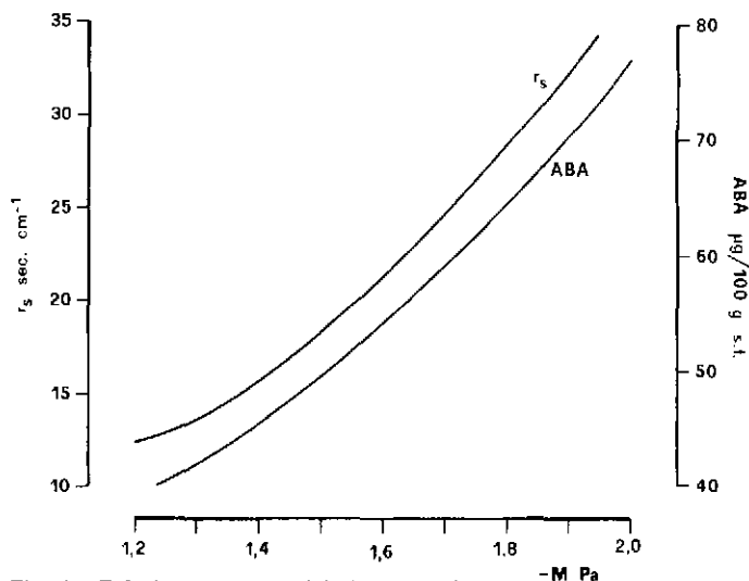
Fig. 1 - Relazioni tra potenziale idrico, resistenza stomatica e livelli fogliari di ABA, in portinnesti sottoposti a stress idrico ( r_s = 17,5 - 26,4 x + 18x^2 , R^2 = 0,95 ; ABA = 37,4 - 27,0 x + 23,4 x^2 , R^2 = 0,92 )
